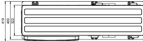
Vista frontale
