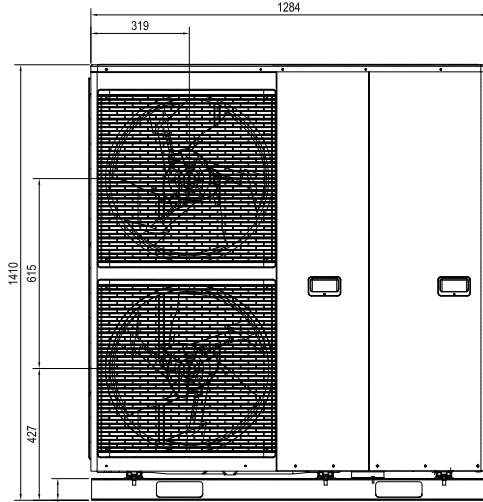
Vista frontale
