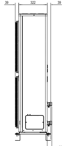
Vista laterale
