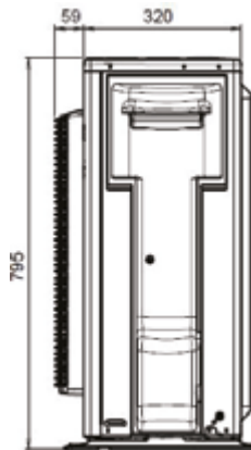
Vista laterale
